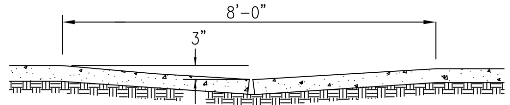
SUNKEN SIDEWALK
